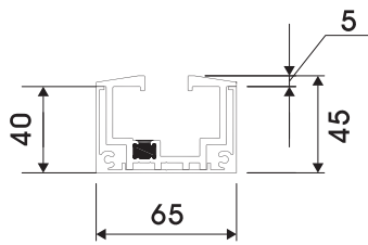
▲ 기본 하부레일 (단열)
