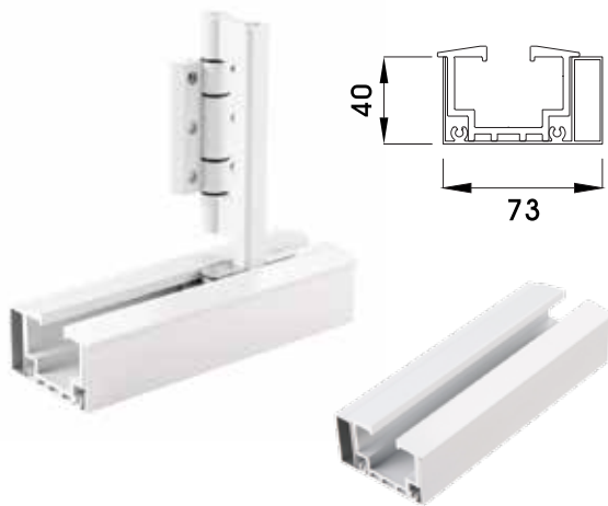
▲ UPVC 용 하부롤러 / 하부레일
