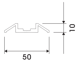
▲ '로우레일' 날개형
