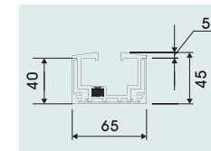
기본 하부레일 (단열)
