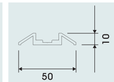
로우레일 매립형(만능커버포함)
