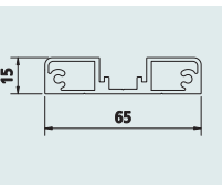
신형오픈레일
